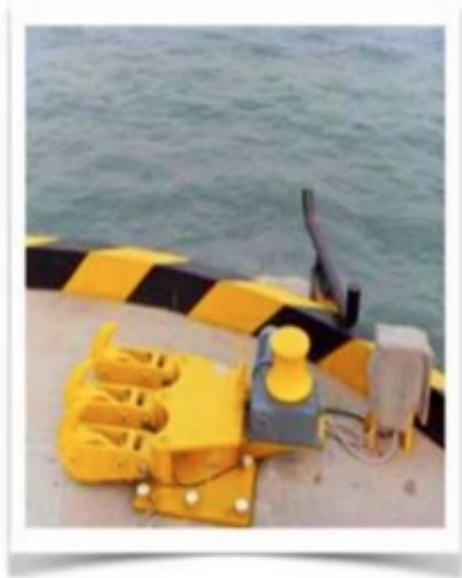
Гак швартовый быстроотдающийся
